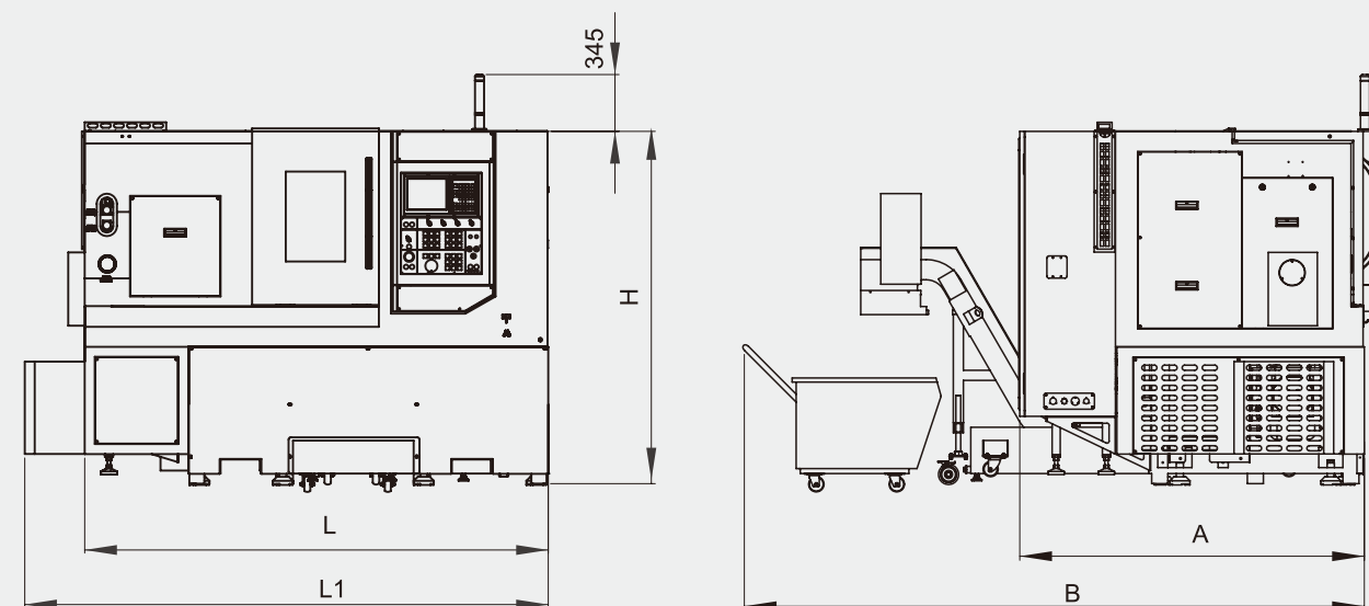
机器外观尺寸图 Machine exterior dimensions diagram
