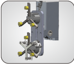
气动摆缸\ 气动手爪集成， 水平对置。
